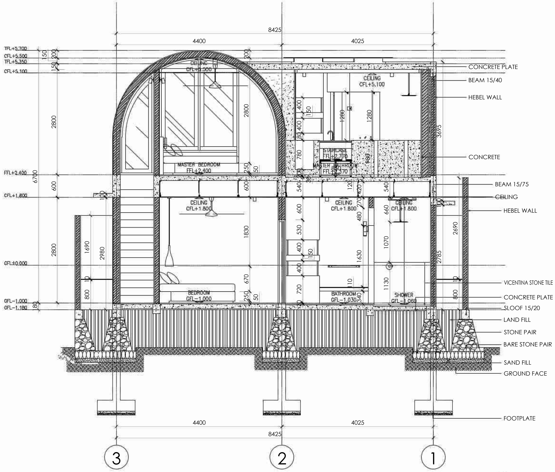
SECTION B-B VILLA B Scale 1 : 50
