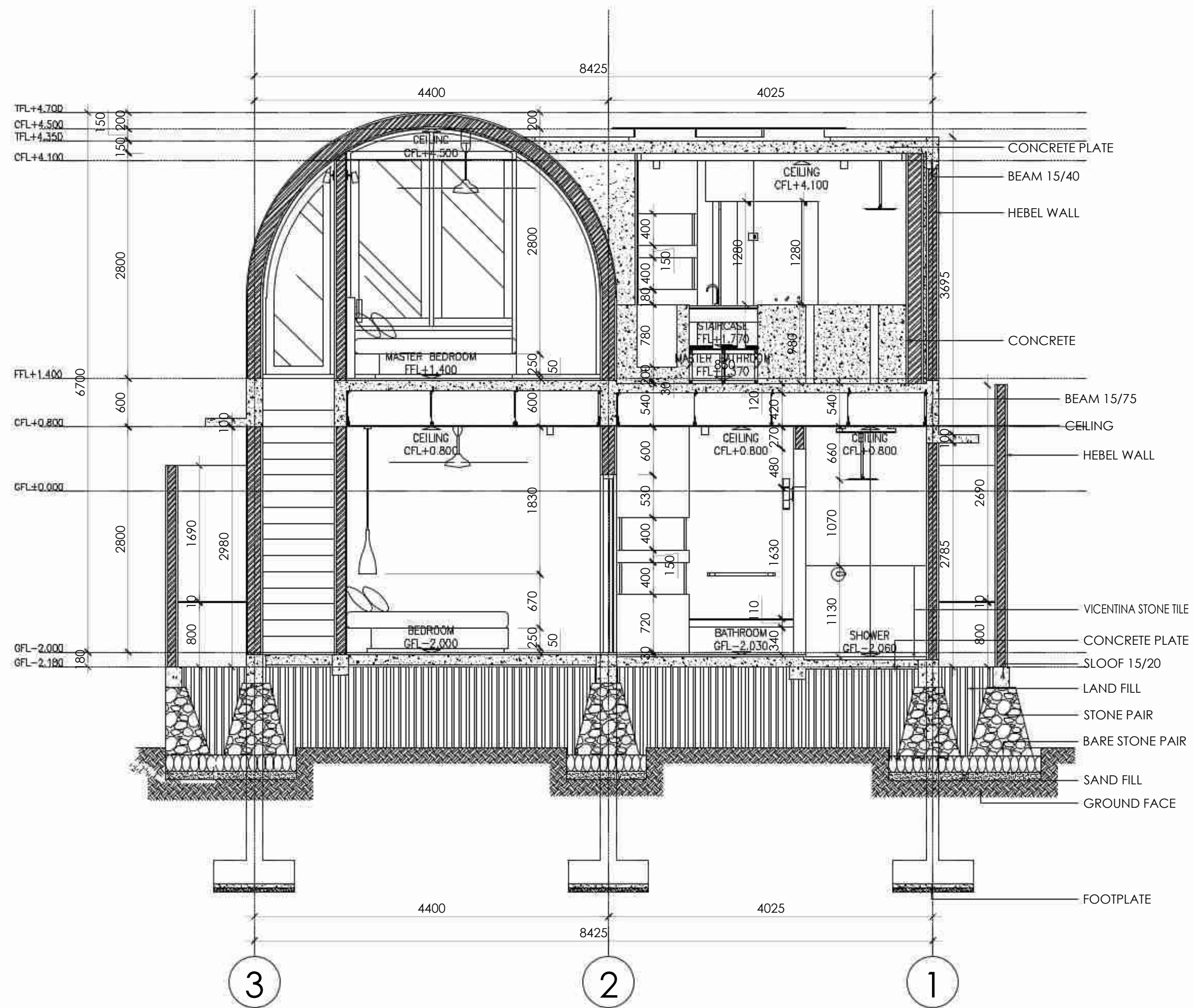
SECTION B-B VILLA A Scale 1 : 50
