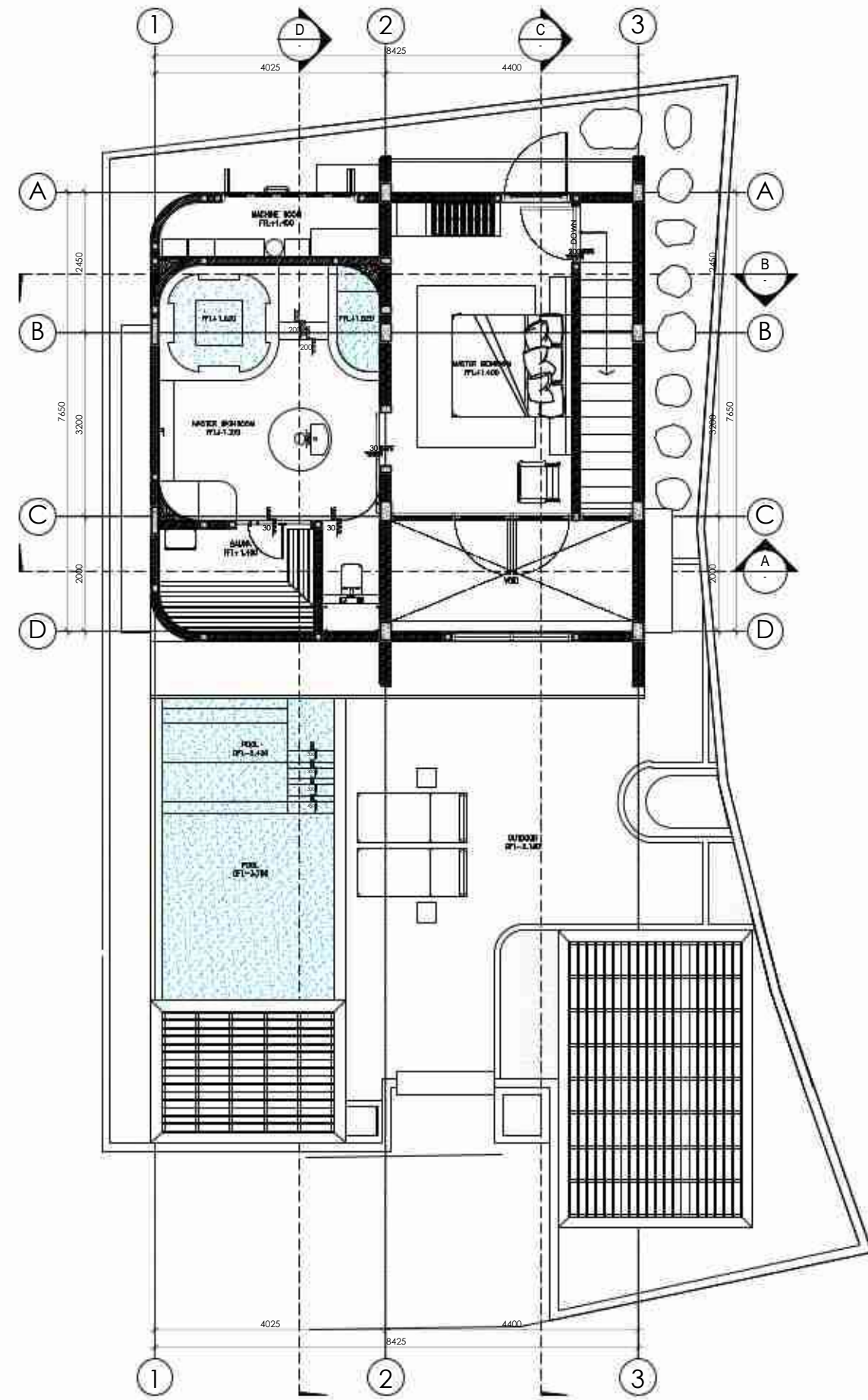
SECTION VILLA A Scale 1 : 100
