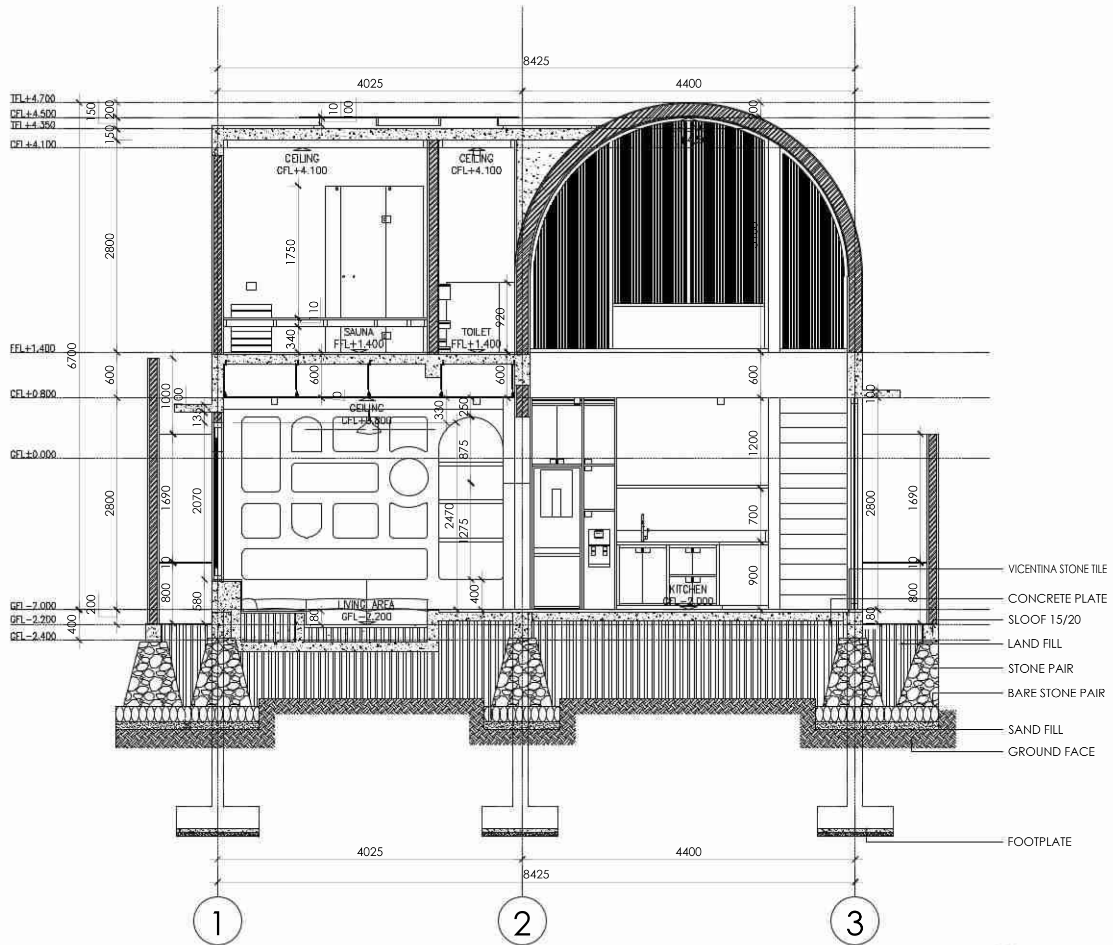
SECTION A-A VILLA A Scale 1 : 50
