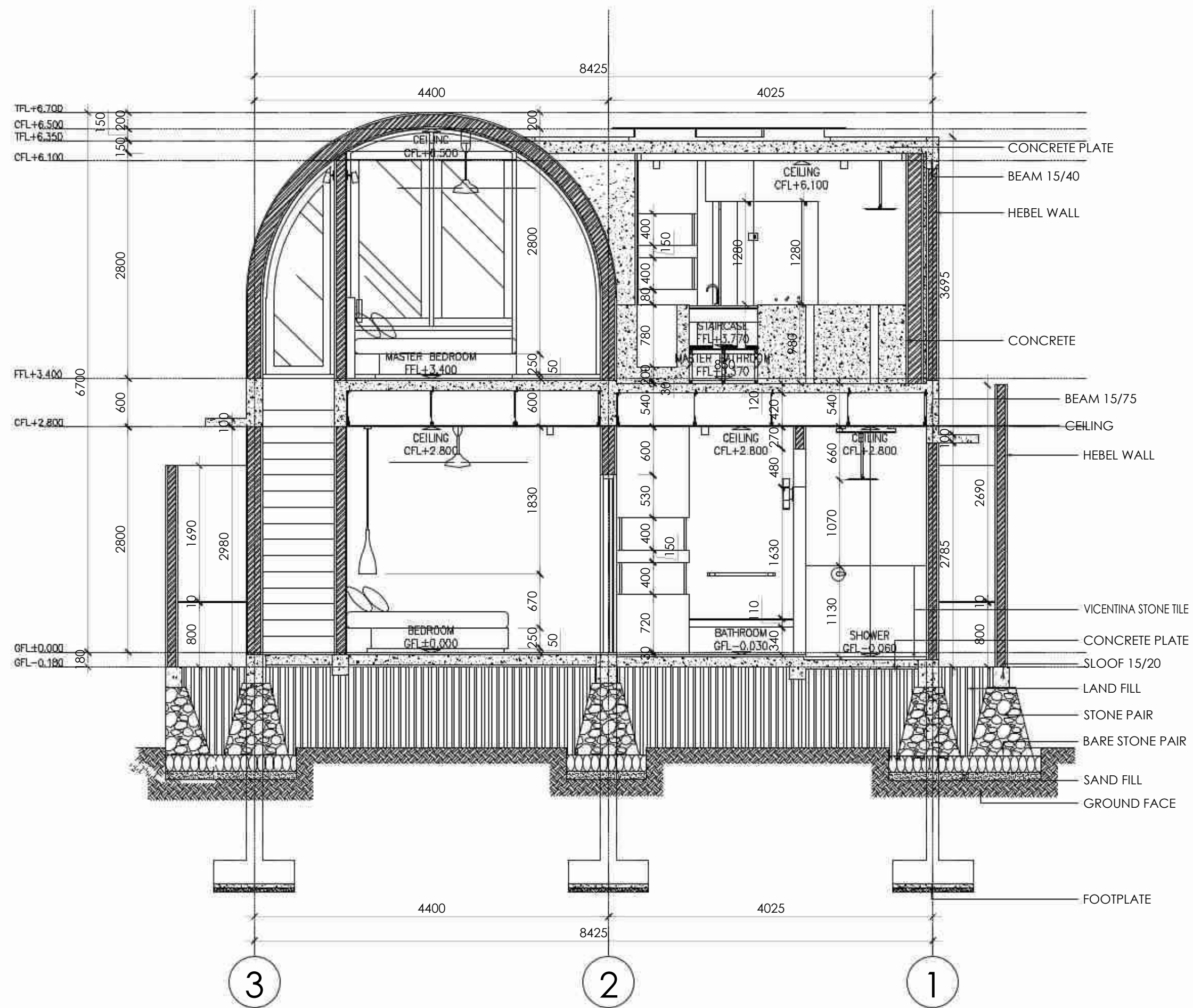
SECTION B-B VILLA C Scale 1 : 50
