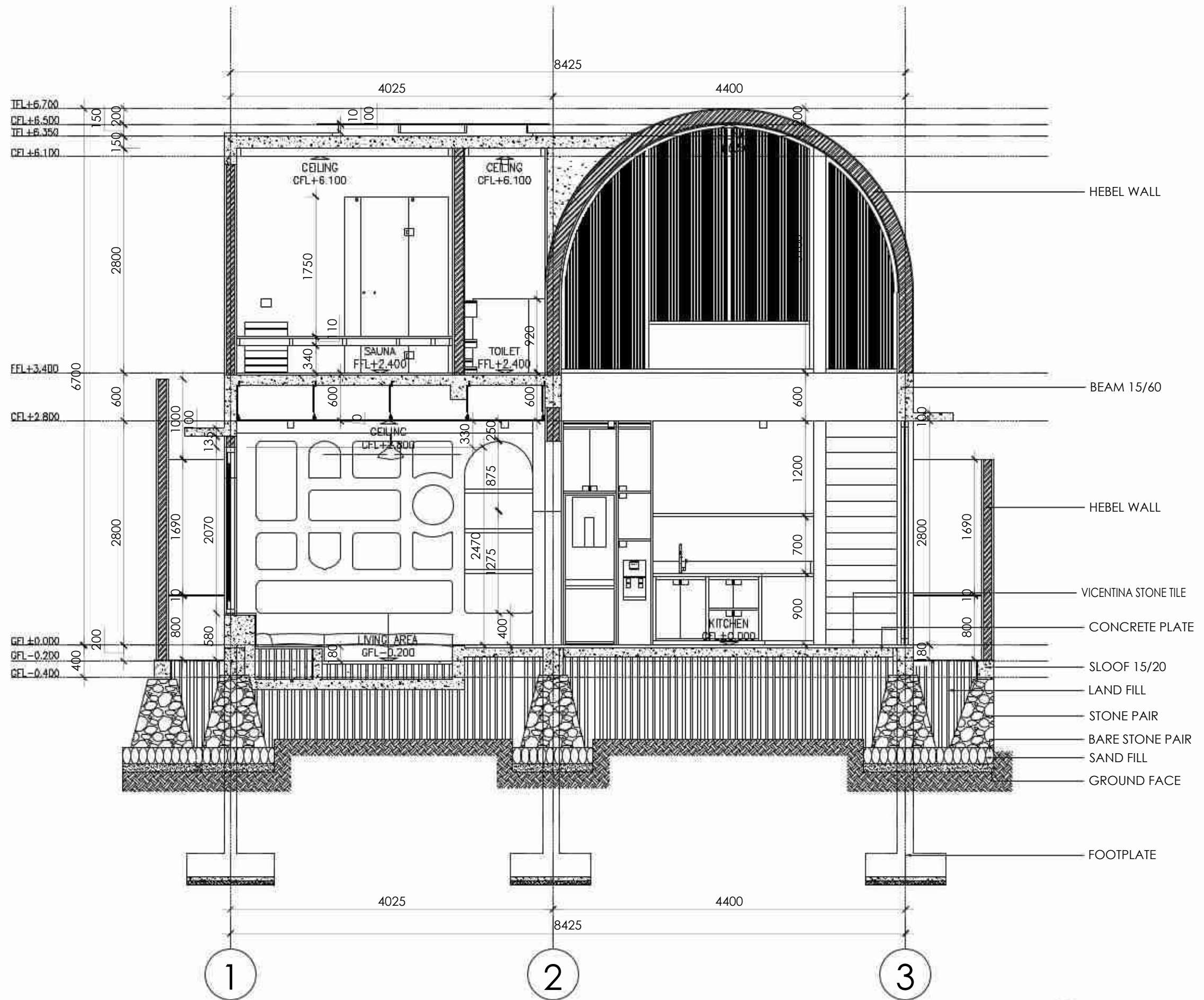
SECTION A-A VILLA C Scale 1 : 50
