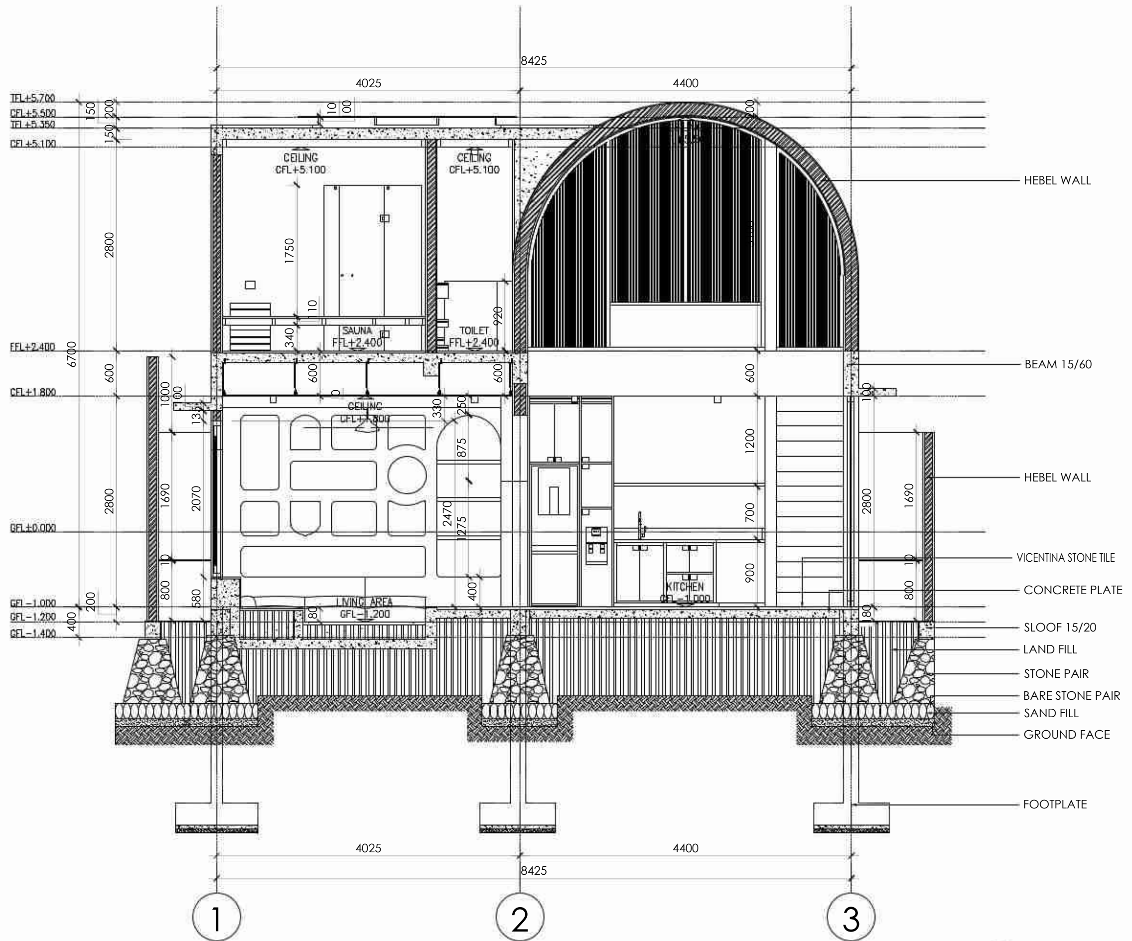
SECTION A-A VILLA B Scale 1 : 50
